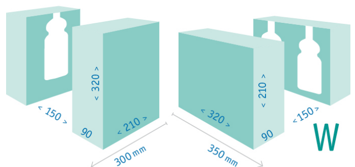
Abmessungen der Form (mm)
